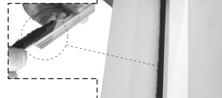
19 Bürsten in Profil einziehen und Profil einkleben
